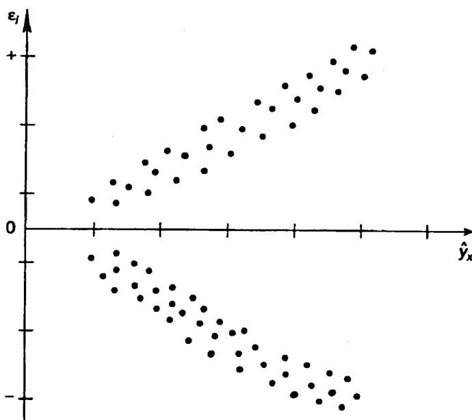
Рис. 2.5. Гетероскедастичность: большая дисперсия \mathcal{E}_i для больших значений \hat{y}_x .
