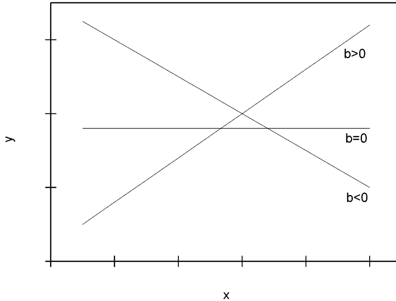
Рис.1.3. Наклон линии регрессии в зависимости от значения параметра b .
