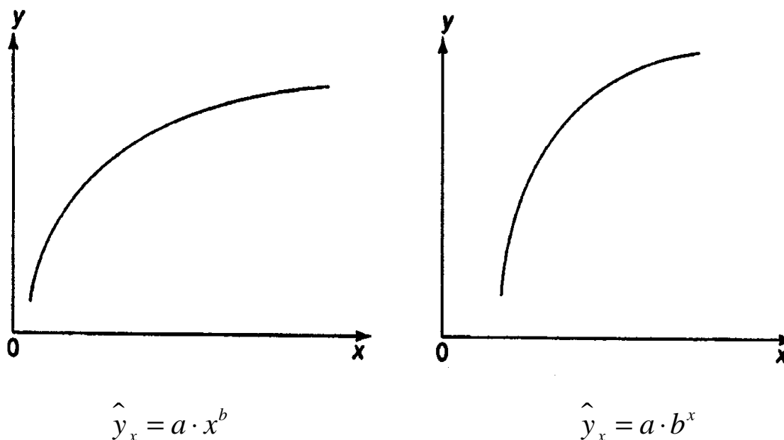
Рис. 1.1. Основные типы кривых, используемые при количественной оценке связей между двумя переменными.
