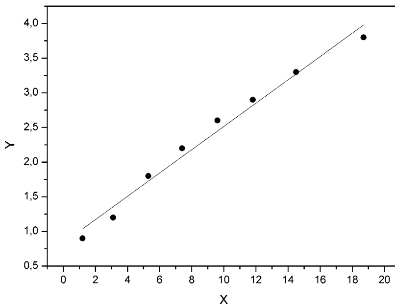
Рис. 1.5. Исходные данные и теоретическая прямая.
